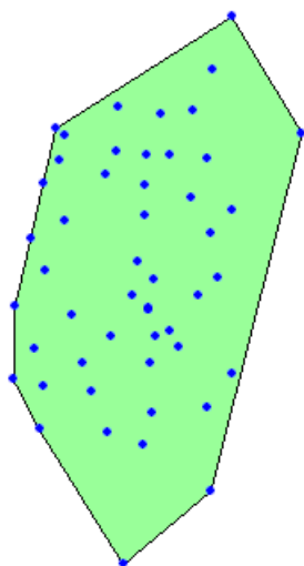
Выпуклая оболочка
