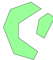
Отсечение
